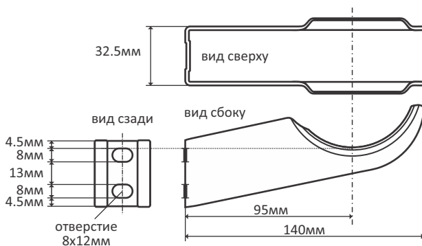
Рисунок 4 - Размеры настенных кронштейнов Unilux
